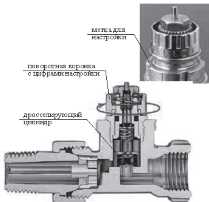
Рисунок 11.14 – Устройство предварительной настройки
