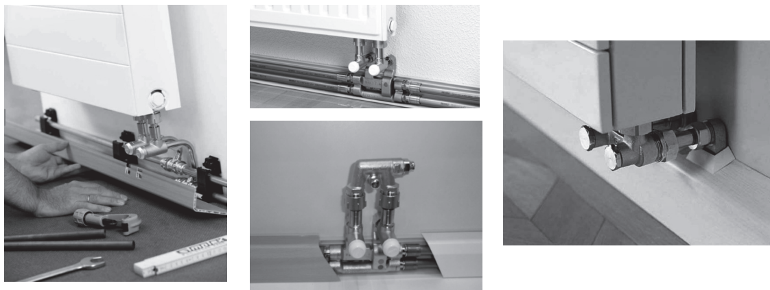
Рисунок 7.5 – Элементы плинтусной системы отопления
