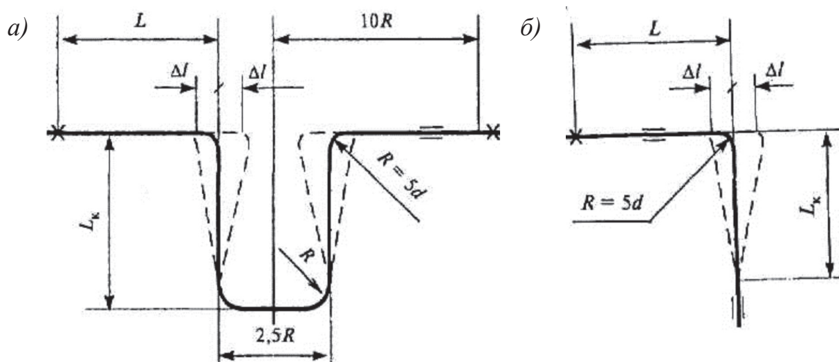
а) – П-образный компенсатор; б) – Г-образный компенсатор
