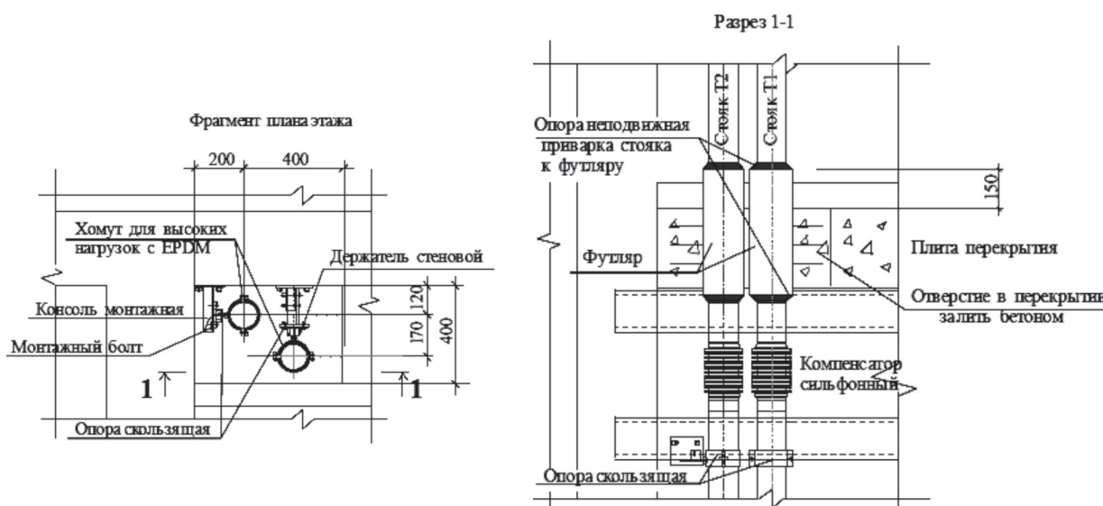
Рисунок 11.2 – Установка сильфонных компенсаторов на стояках системы отопления
