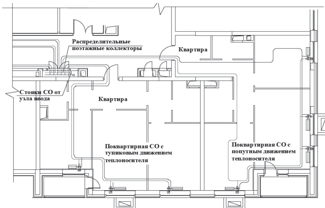
Рисунок 7.1 – Схема двухтрубной поквартирной (горизонтальной) СО
