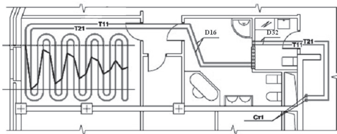
Рисунок 7.4 – Схема системы напольного отопления с параллельной укладкой греющих труб в виде двойного змеевика
