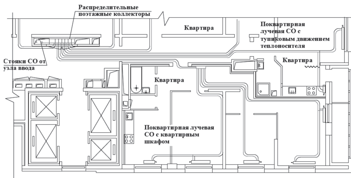
Рисунок 7.2 – Схема двухтрубной лучевой поквартирной (горизонтальной) СО
